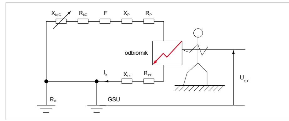
Rys. 12. Metodyka wyznaczenia przekroju przewodu ochronnego S_{PE} łączącego chronione urządzenie z GSU, dla spełnienia warunku U_{ST} \leq U_L [10]
