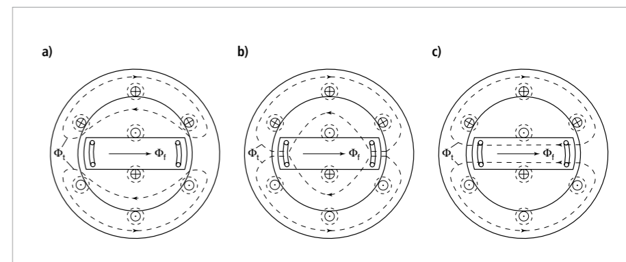
Rys. 8. Przebieg wypchanego poza wirnik strumienia stojana [10]: a) stan podprześciowy, b) stan przejściowy, c) stan ustalony
