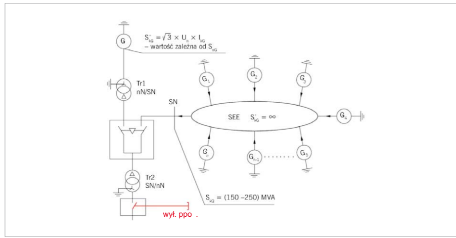
Rys. 11. Porównanie mocy zwarciowych SEE i zespołu prądowłórczego [10]
