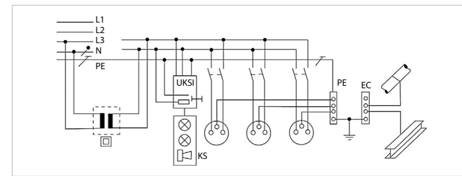
Rys. 7. Schemat instalacji poż. zasilanej w układzie IT [10], gdzie: UKSI – układ kontroli stanu izolacji (reagujący na zmniejszenie się poziomu izolacji poniżej 50 k \Omega ), z przyciskiem kontrolnym, KS – kasetka ze wskaźnikiem świetlnym i akustycznym (lampka zielona – stan prawidłowy, lampka pomarańczowa i brzęczyk – stan awaryjny), PE – przewód ochronny – szyna połączeń ochronnych urządzeń elektrycznych, EC – szyna połączeń wyrównawczych
