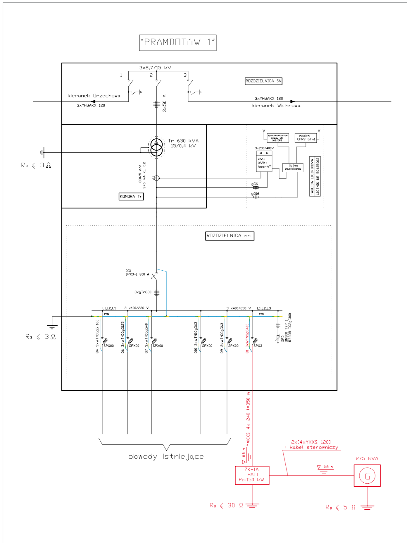
Rys. 2. Schemat ideowy stacji TR 15/0,4 kV „Pramdotów 1”
