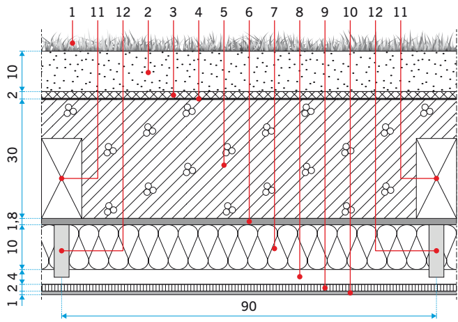
RYŚ. 6. Wariantowe rozwiązania materiałowe stropodachów pełnych z zastosowaniem materiałów ekologicznych: ocieplenie stropodachu od wewnątrz grubości 10 cm (wariant II); rys.: [2]
