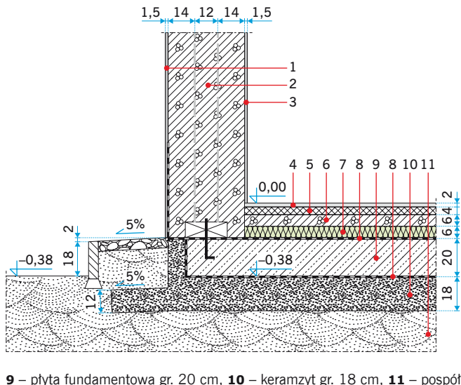
RYS. 9. Wariantowe rozwiązania materiałowe przegród stykających się z gruntem: izolacja podłogi na gruncie/plyta z pianki poliuretanowej grubości 6 cm (wariant II); rys.: [2]
