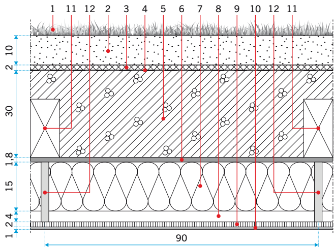
RYŚ. 7. Wariantowe rozwiązania materiałowe stropodachów pełnych z zastosowaniem materiałów ekologicznych: ocieplenie stropodachu od wewnątrz grubości 15 cm (wariant III); rys.: [2]
