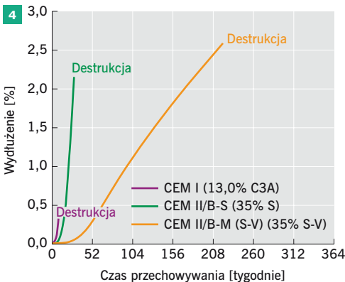
rys. 2-5. Zmiany liniowe zapraw cementowych wykonanych z różnych cementów przechowywanych przez 7 lat w roztworze \text{Na}_2\text{SO}_4 : cementy popiołowe (2), cementy żużlowe (3), cementy popiołowo-żużlowe (4) i cementy wapienne (5); rys.: [18]
