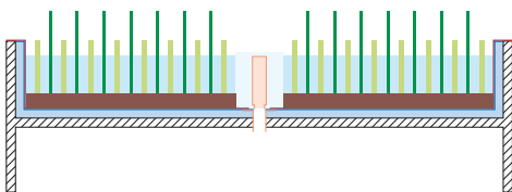
RYS. 7. Dach bagienny; rys.: [12]
