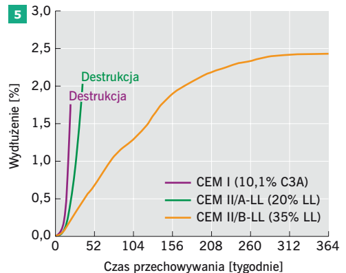
rys. 2-5. Zmiany liniowe zapraw cementowych wykonanych z różnych cementów przechowywanych przez 7 lat w roztworze \text{Na}_2\text{SO}_4 : cementy popiołowe (2), cementy żużlowe (3), cementy popiołowo-żużlowe (4) i cementy wapienne (5); rys.: [18]
