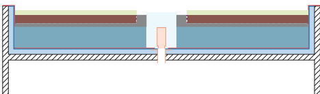
RYS. 6. Dach zielony z drenażem magazynującym; rys.: [12]
