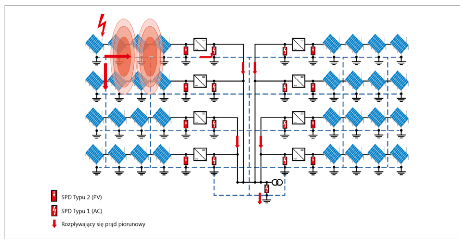
Rys. 10. Ochrona przeciwprzebieciowa farmy fotowoltaicznej z falownikami przeznaczonymi dla każdej gałęzi (z oznaczonym możliwym do wystąpienia rozpływającym się prądem doziemnego wyładowania piorunowego) rys. J. Wiater
