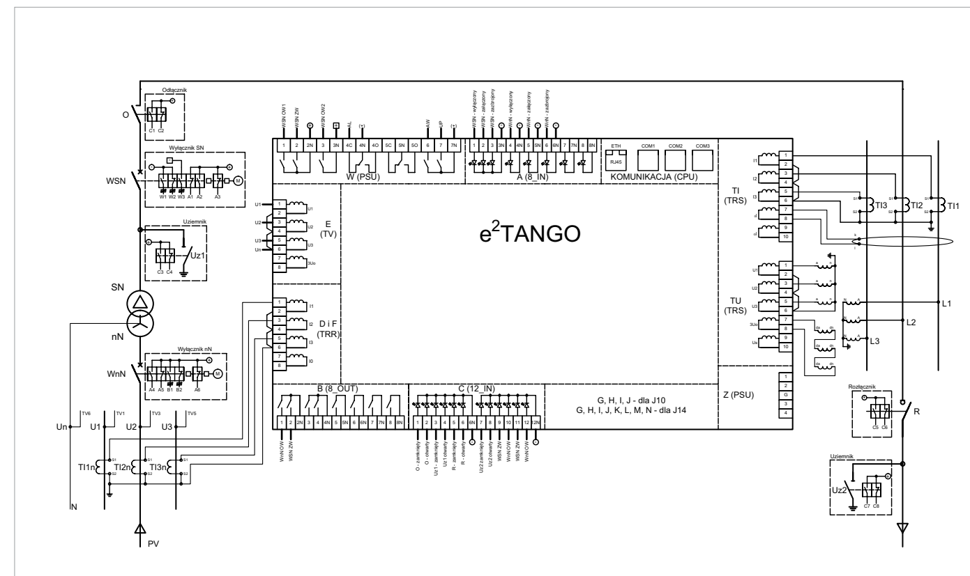
Rys. 3. Schemat aplikacyjny sterownika zabezpieczeniowego e 2 TANGO realizującego funkcje zabezpieczeniowe, pomiary prądu i napięcia, sterowania – zarówno po stronie SN jak i nn transformatora
