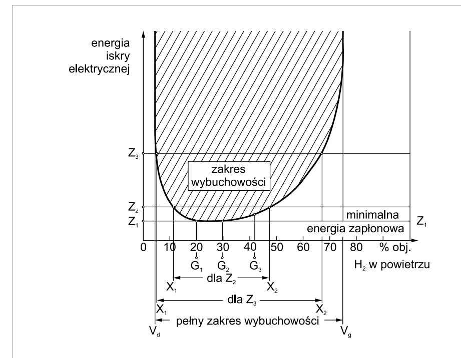
Rys. 11. Zależność energii zapłonowej od składu mieszanin wodoru z powietrzem, gdzie: Z_1 – minimalna energia zapłonu E_{\text{min}} = 0,019 \text{ mJ} , V_d – dolna granica wybuchowości (DGW), V_g – górna granica wybuchowości (GGW) [4]
