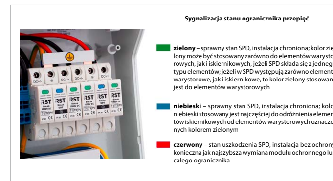
Rys. 5. Sygnalizacja stanu SPD
