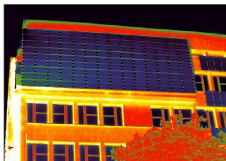
Fot. 6. Prawidłowo wykonane zdjęcie termowizyjne [7]
