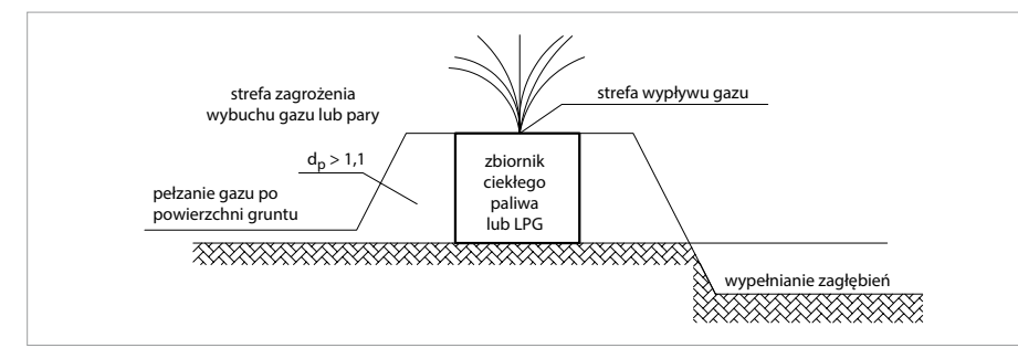
Rys. 4. Zachowanie się oparów paliwa ciekłego cięższego od powietrza rys. J. Wiatr
