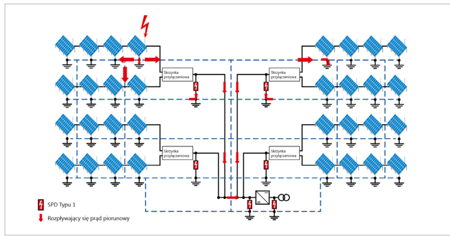
Rys. 9. Ochrona przeciwprzebieciowa farmy fotowoltaicznej z falownikiem centralnym (z oznaczonym możliwym do wystąpienia rozpływającym się prądem doziemnego wyładowania piorunowego) rys. J. Wiater
