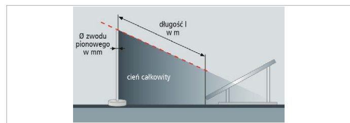
Rys. 7. Odstęp paneli PV od zwodu pionowego zapewniający eliminację cienia zupełnego [2]
