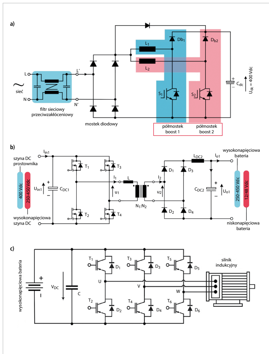
Rys. 3. Schemat blokowy przetworników ładowarki pokładowej i DC/DC: a) jednofazowa AC/DC w topologii PFC, b) izolowany przetwornik DC/DC z jednokierunkową konfiguracją PSFB, c) półmostkowy falownik trójfazowy do napędu silnika prądu przemiennego (napęd główny pojazdu EV) rys. M. Żurek-Mortka, J. Szymański
