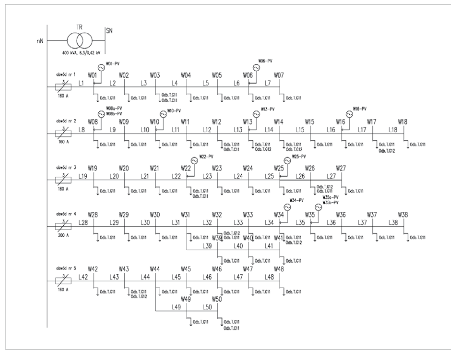
Rys. 1. Model sieci niskiego napięcia w wariancie 1 rys. J. Traskiewicz, M. Przygodzki
