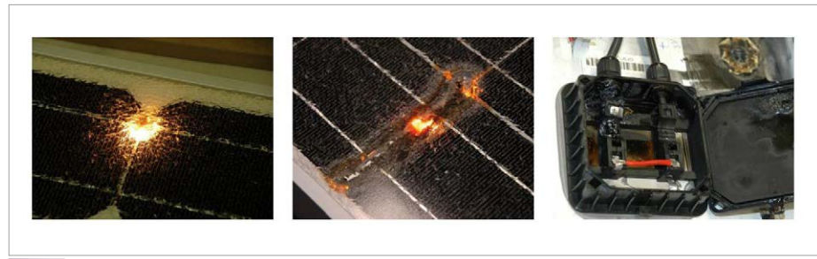
Rys. 7. Wizualizacja łuków elektrycznych oraz ich skutków w instalacji PV [19]
