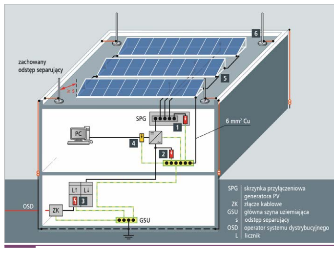
Rys. 5. Budynek z zainstalowaną instalacją piorunochronną spełniającą wymagane odstępsej izolacyjne: 1 – wejście DC falownika, 2 – strona AC falownika, 3 – sieć zasilająca nn 230/400V, 4 – interfejs przesyłu danych, 5 – połączenia wyrównawcze/zaciski uziemiające, 6 – układ zwodów pionowych na dachu/iglica odgromowa z podstawą betonową [2]
