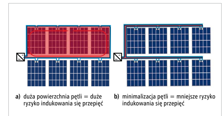
Rys. 6. Pętle powstające w obwodach DC instalacji PV
